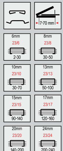
BOXER 5500 PREMIUM heavy duty stapler nagytehetsítményű fűzőgép
